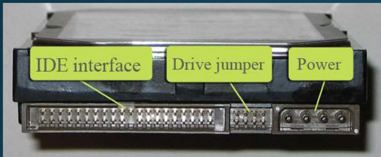
IDE / PATA
