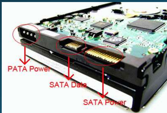
SATA
